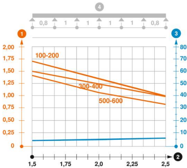
Diagrama de carga bandeja portacables MKSM 85
