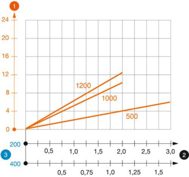
Diagrama de carga soporte en U tipo US 3 K
